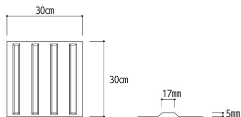
【図9.1】 種類（JIS T 9251による 資料編（各種規格等）資-112～115 参照）
