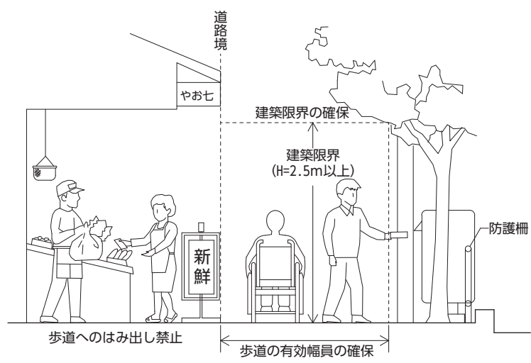
【図2.1】有効幅員の考え方
