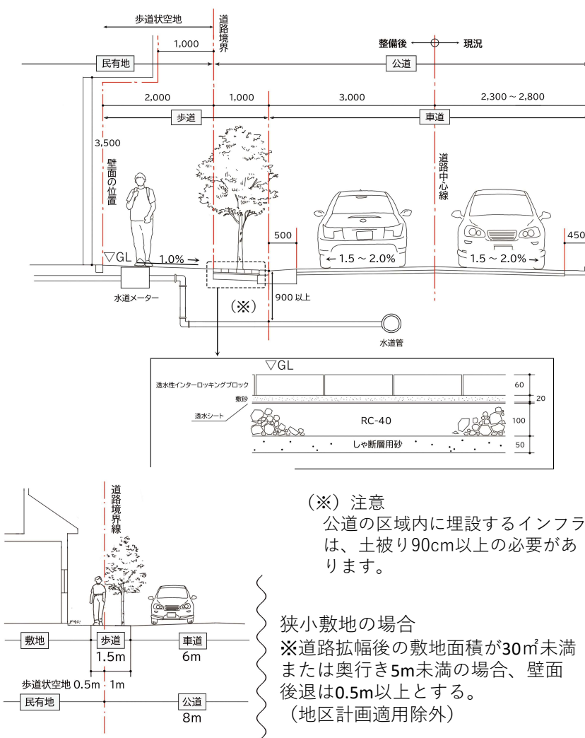
図4 | 若葉通りと区画道路3号の断面図 ～標準的な例～
