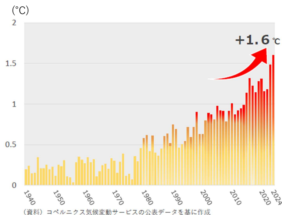
産業革命前頃の平均気温と各年の気温との差
