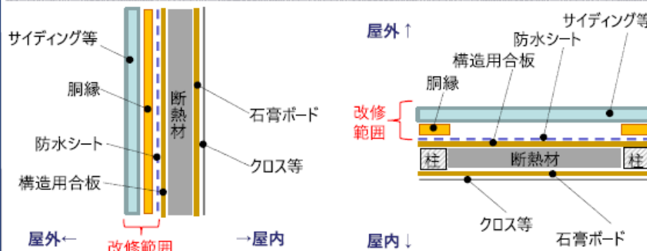
図1-1 横から見た断面図
