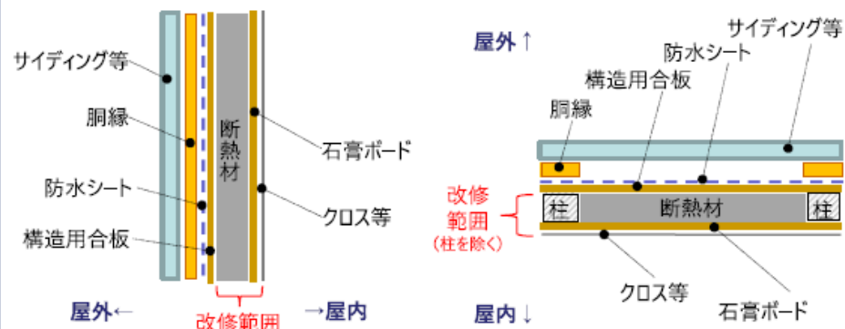
図2-1 横から見た断面図
