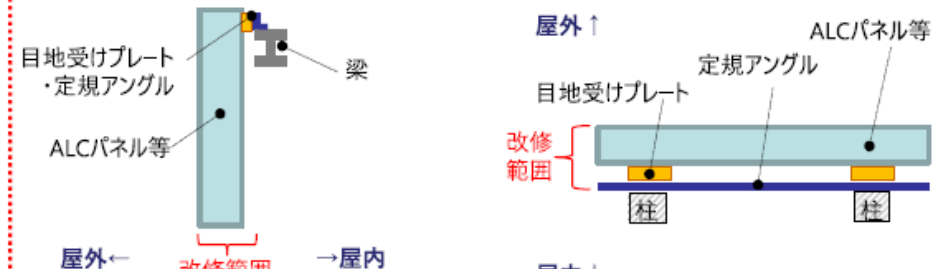
図1-7 横から見た断面図
