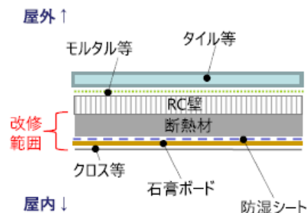
RC造（壁式構造・内断熱の場合）
