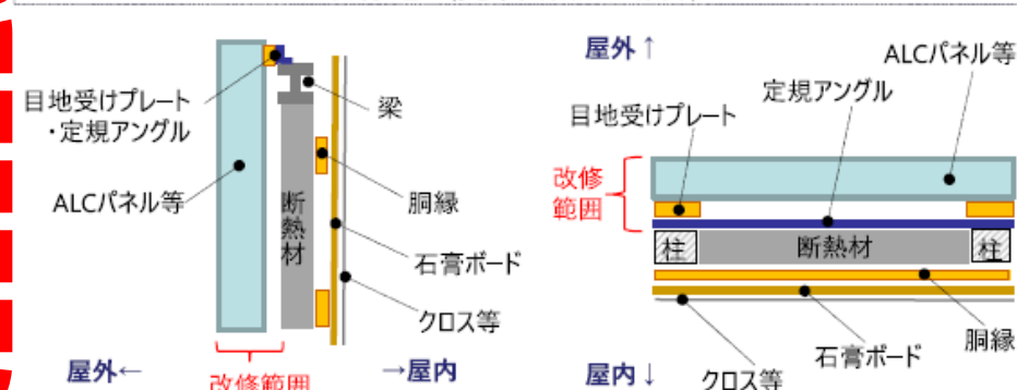
図1-3 横から見た断面図
