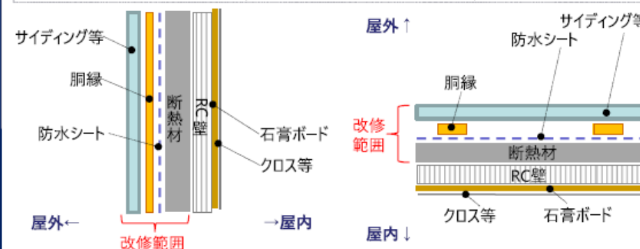
図1-5 横から見た断面図
