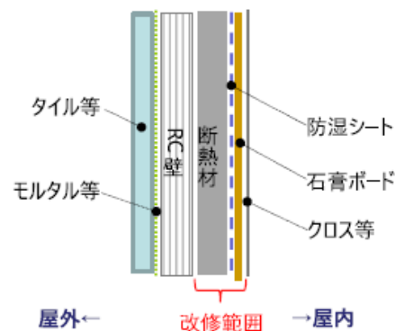
図2-5 横から見た断面図
