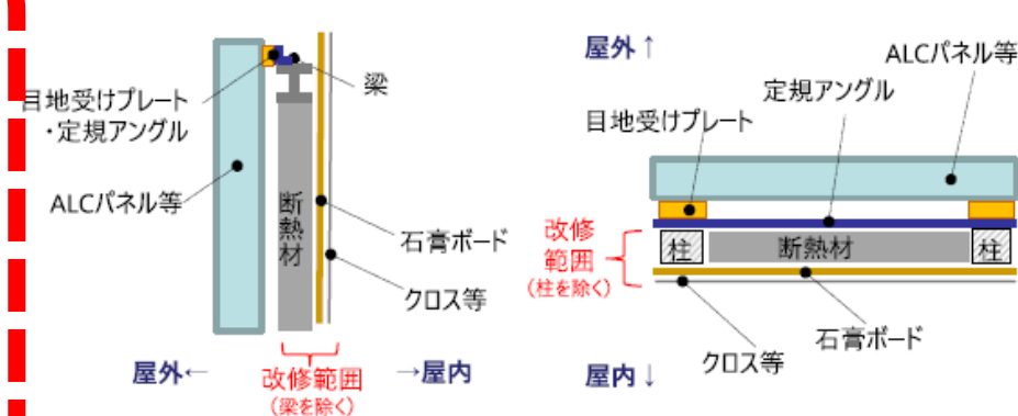
図2-3 横から見た断面図
