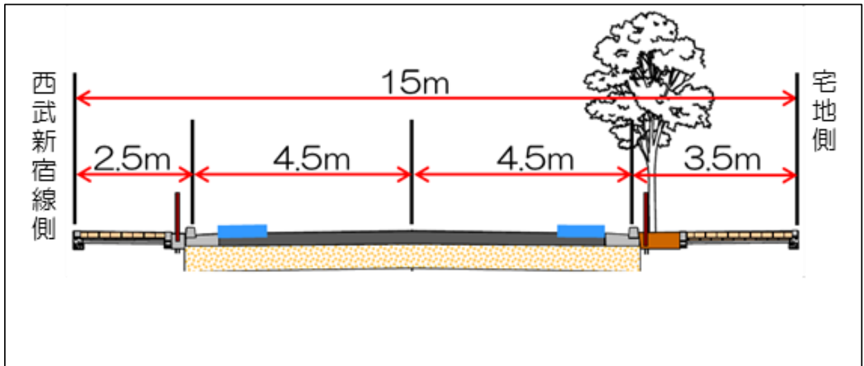
標準横断面図 ～ I 期区間～
