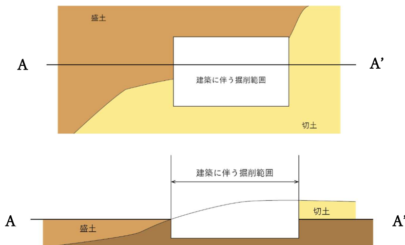
図 8 建築に伴う掘削範囲
