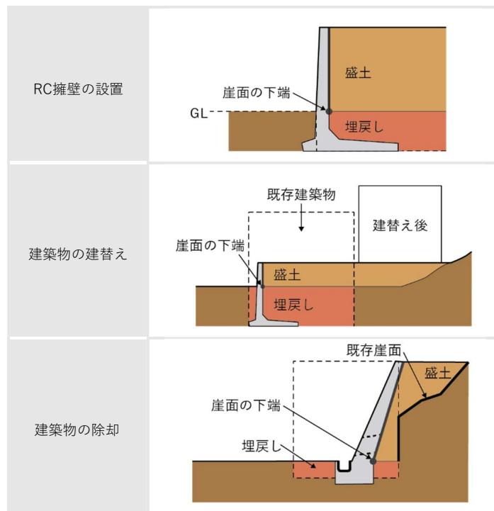
図 3 盛土と埋戻し
