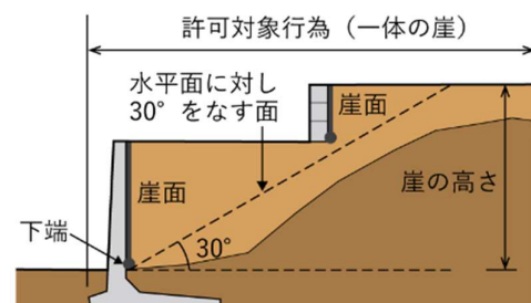
図 4-2 崖の高さ（一体の崖）
