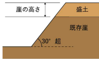
図2-1 崖の高さ（盛土）
