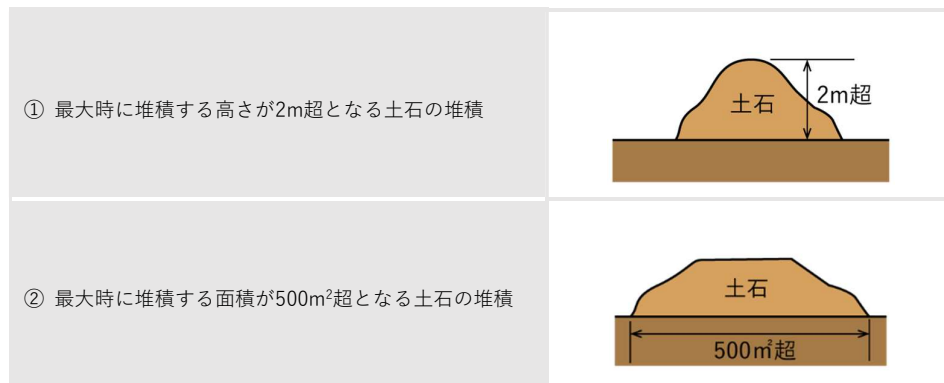
図5 許可を要する工事（土石の堆積）
