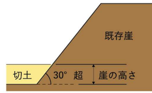
図2-2 崖の高さ（切土）
