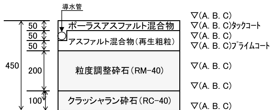
排水性型 45型
