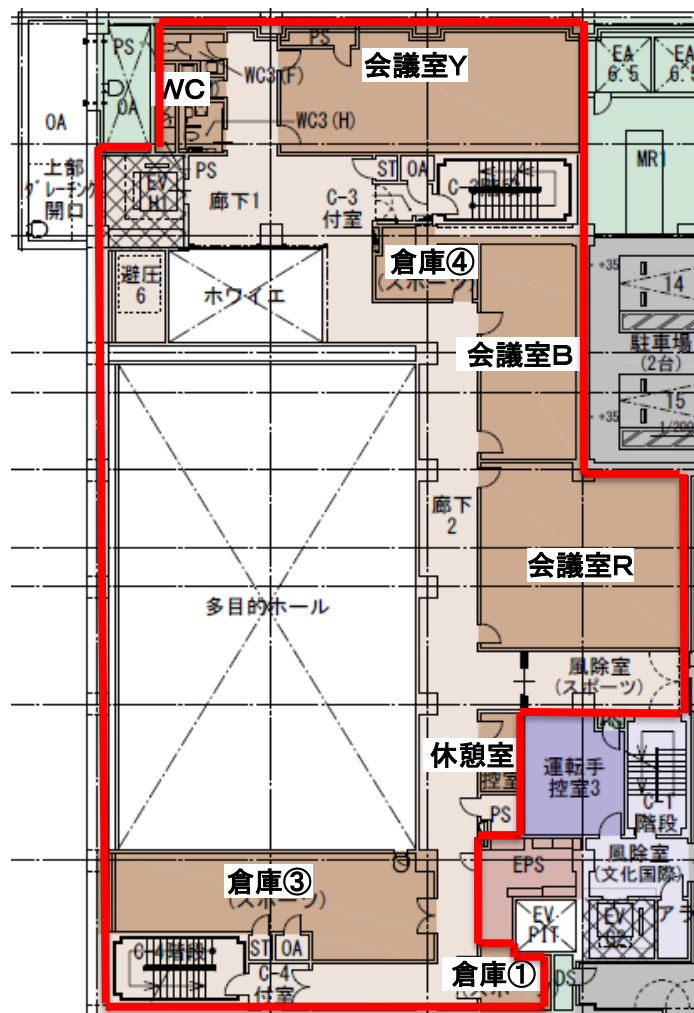
B1階平面図
