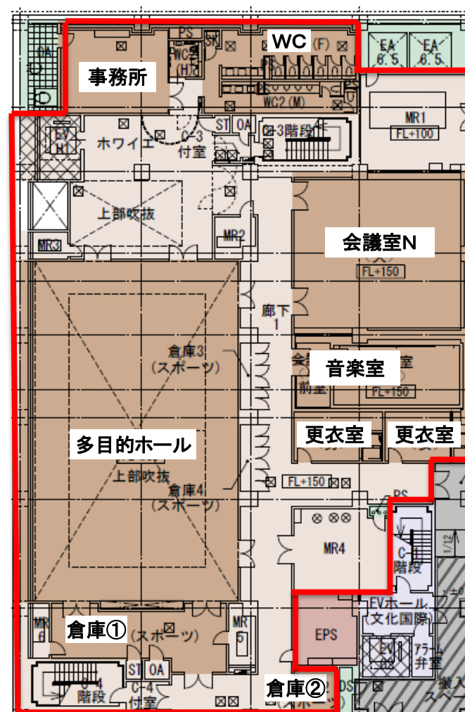
B2階平面図
