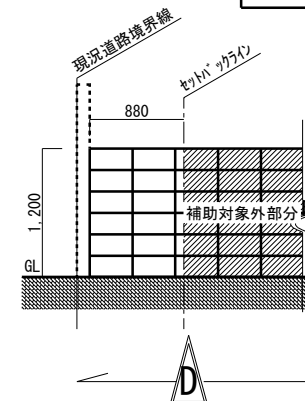
立面図
