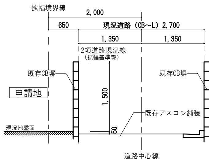
B-B' 断面
