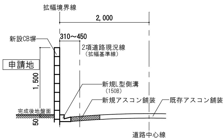
A-A' 断面
