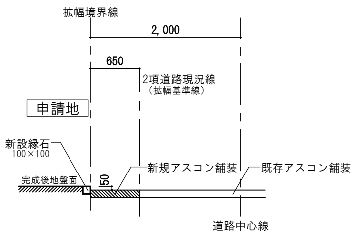
B-B' 断面
