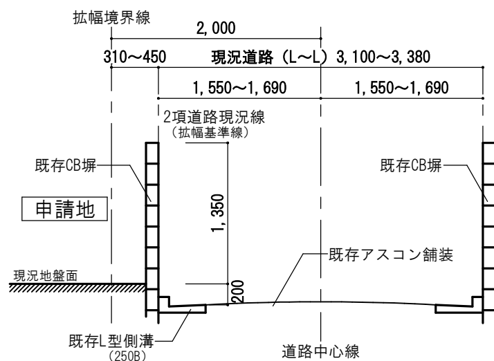
A-A' 断面
