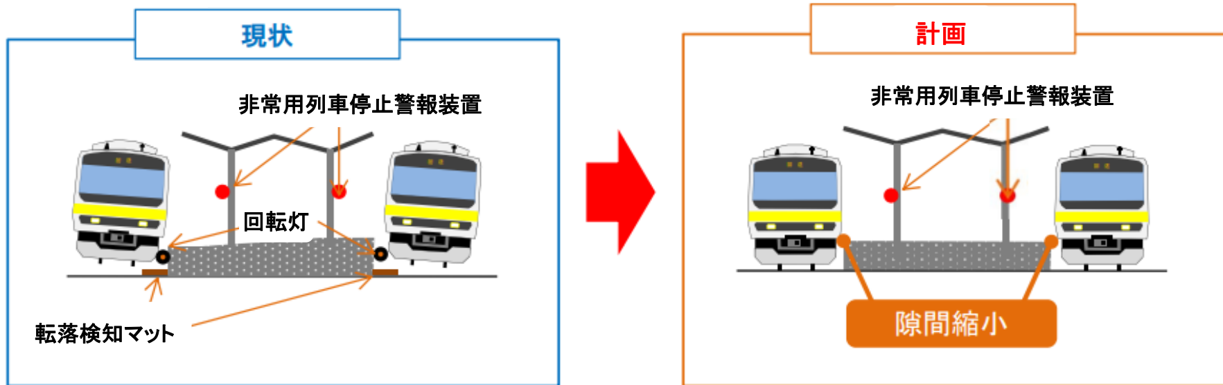
【ホーム断面イメージ図】
