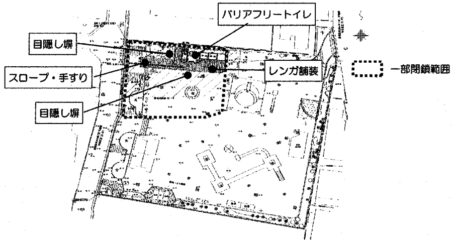
完成予想平面図
