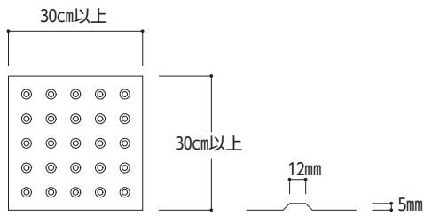
【図14.4】 種類 (JIS T 9251による 資料編 (各種規格等) 資-102~105 参照)
