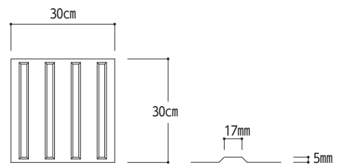
【図14.4】 種類 (JIS T 9251による 資料編 (各種規格等) 資-102~105 参照)
