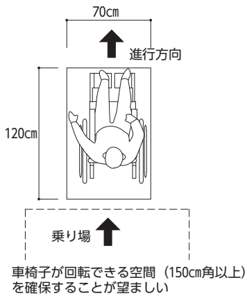
【図7.3】 籠の大きさ
