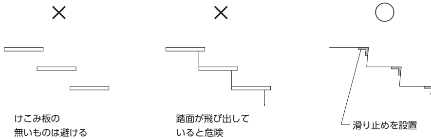
【図4.4】 蹴上げ、路面の形状（つまずきにくい構造の例）
