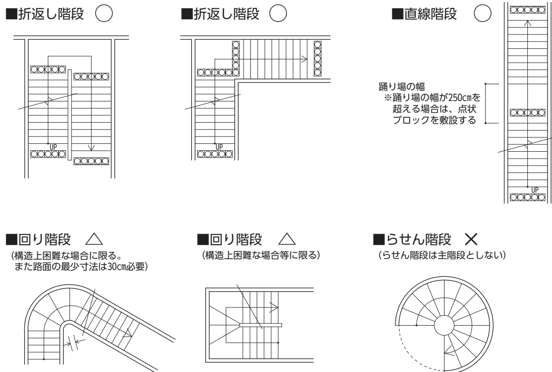
【図4.6】 階段の形状
