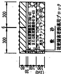
(注) ( ) 表示は乗入れ部舗装D型の寸法を示す。
