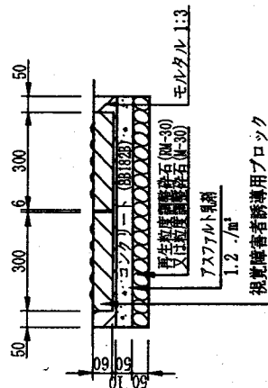
(一般部) S=1/20
