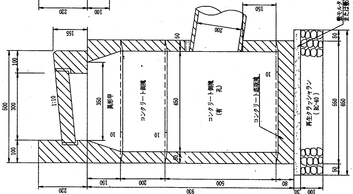
B-B 断面図
